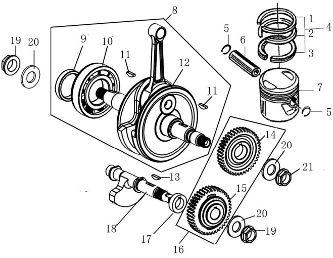
曲轴连杆部件 / 活塞 CRANKSHAFT CONNECTING-ROD ASSY/PISTON
