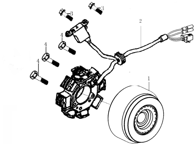
磁电机总成 MAGNETO COMP
