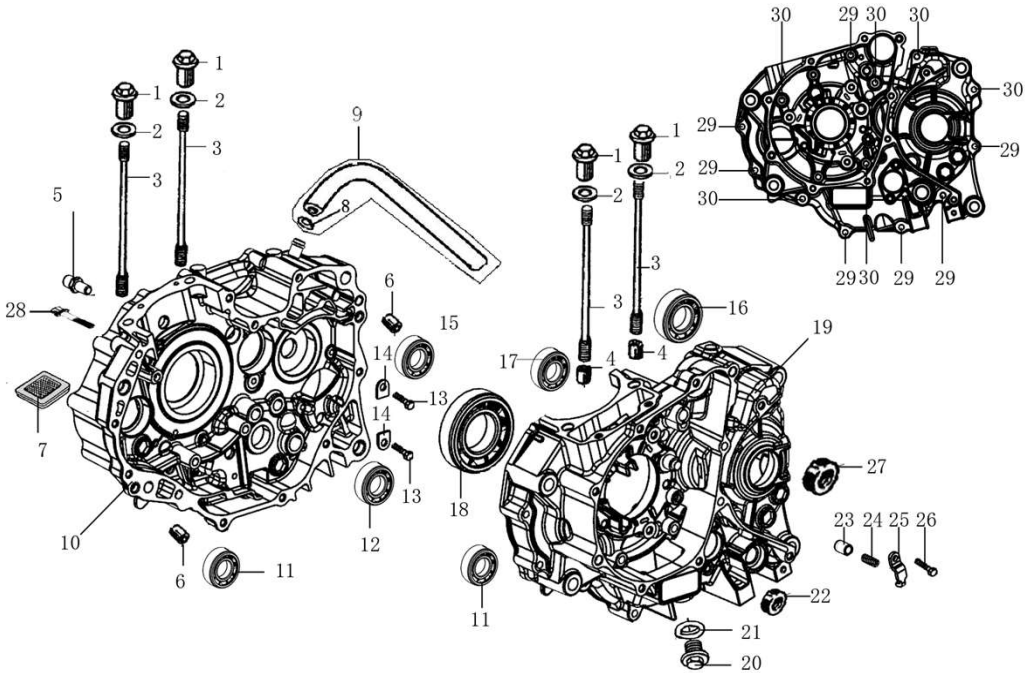
曲轴箱 CRANKCASE
