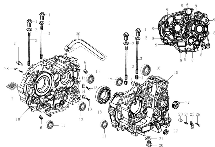
曲轴箱 CRANKCASE
