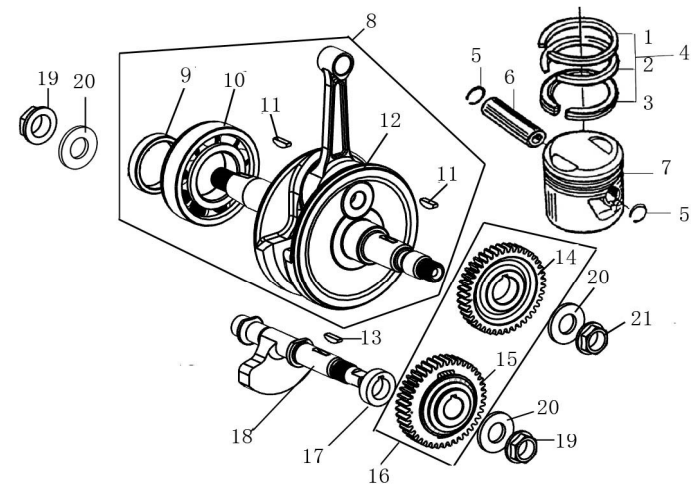
曲轴连杆部件 / 活塞 CRANKSHAFT CONNECTING-ROD ASSY/PISTON
